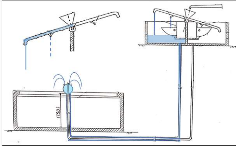
(الشكل 15) مخطط لعمل فوارة الجزري الأولى المتناوبة (الرفاعي، 2000، 232) يلاحظ عملية تبديل اتجاه أنبوب الماء الأفقي المتأرجح لـ (تخرج على شكل ست أقواس) (بتصرف)
