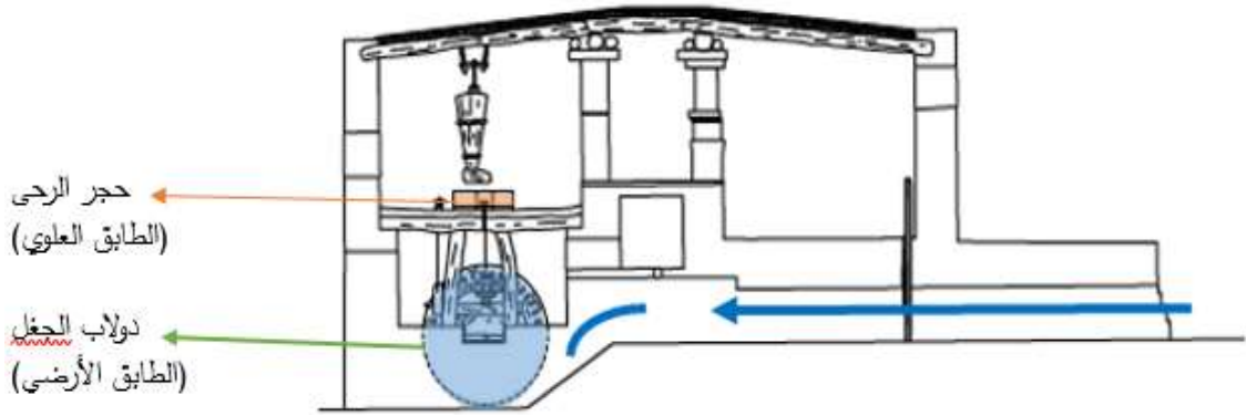
(الشكل 7) توضيح آلية تشغيل وحركة الطاحونة الجغلية، خط سير الماء بشكل منحدر نحو دوليب الجغل (McPhillips, 2016, 152) (بتصرف)
