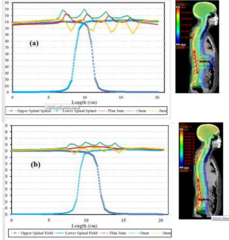
الشكل (6): تأثير عدم الدقة في وضعية المريض بمقدار \pm 3\text{mm} على توزيع الجرعة في التقنية التقليدية (a) والتقنية الجديدة (b) على امتداد 20 cm من PTV تشمل منطقة الاتصال SSJ
