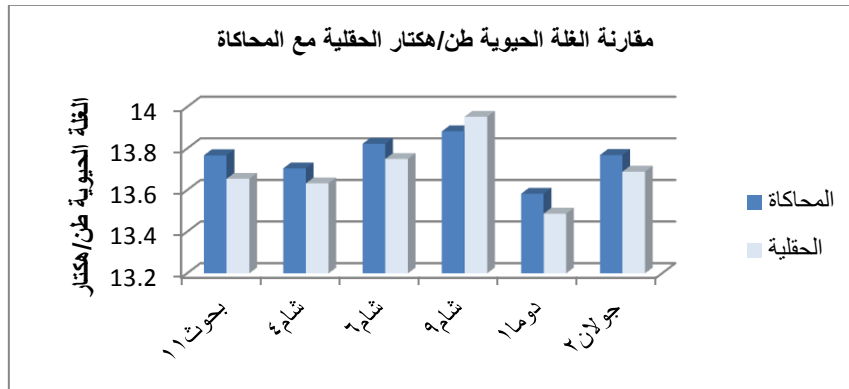
الشكل رقم (4) مقارنة الغلة الحيوية المقاسة حقلياً لأصناف القمح المزروعة مع تلك الناتجة عن المحاكاة باستخدام النموذج الرياضي للموسم 2015-2016
